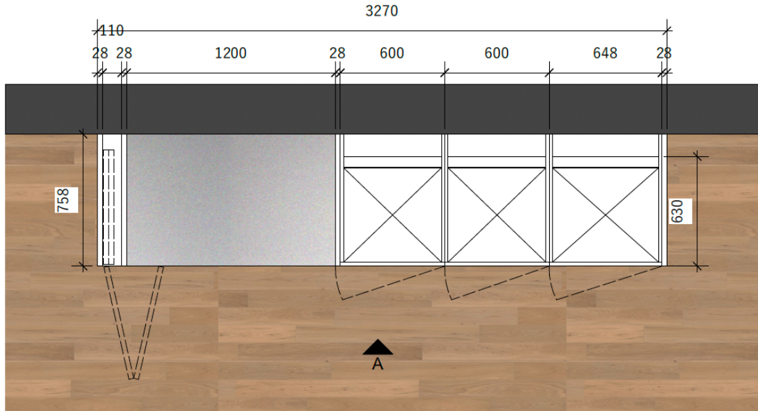
GRUNDRISS
